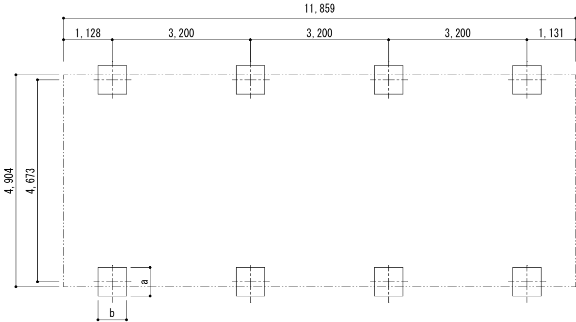
■基礎配置図
